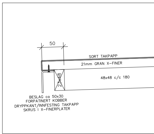
DETALJ 1 - 1:5
